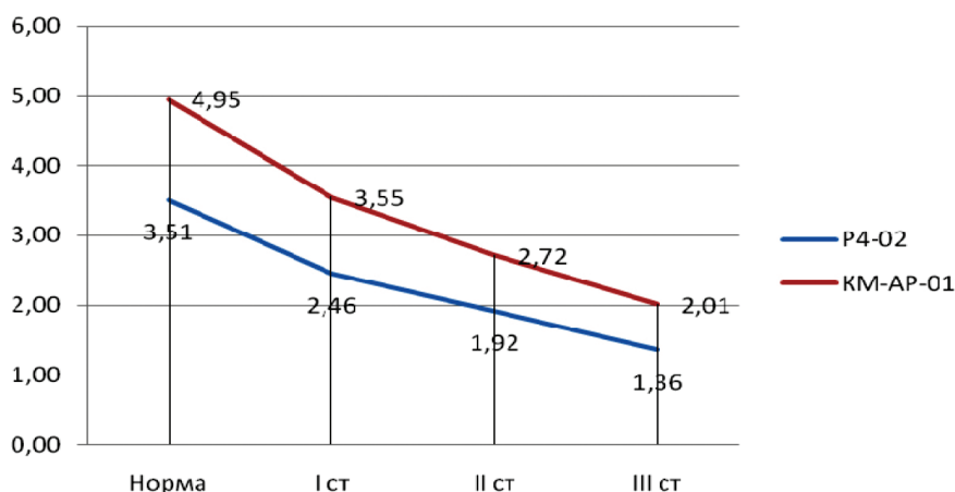
РИС. 7. ДИНАМИКА ИЗМЕНЕНИЯ УдК ПРИ ИСПОЛЬЗОВАНИИ РАЗЛИЧНЫХ РЕОГРАФОВ
